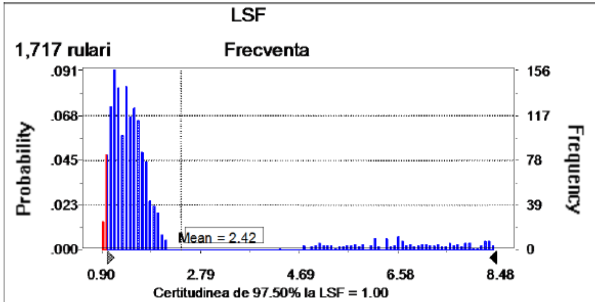
Figura nr. 4.28. Probabilitatea de avarie conducta în zona "b" la timpul "0"
