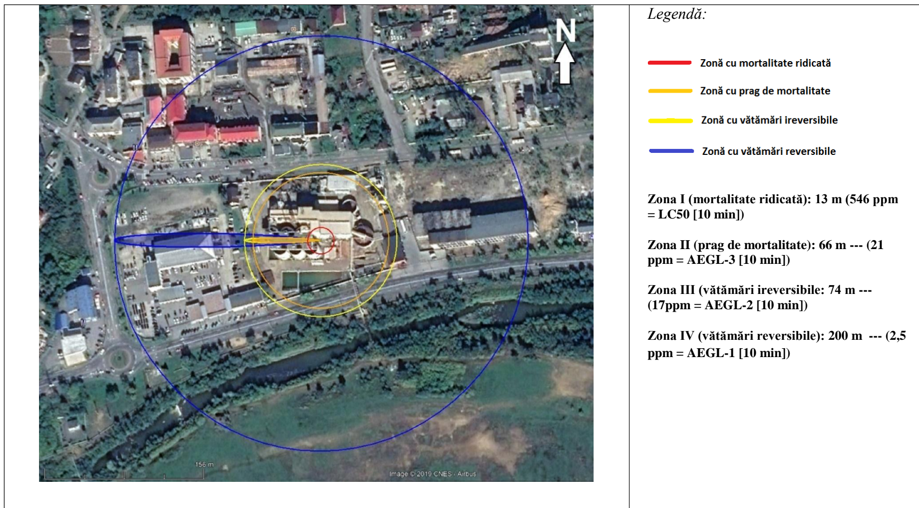
Figura nr. 4.21. Contururi de concentrații de acid cianhidric în cazul emisiei accidentale din reactorul DETOX – condiții meteo nefavorabile
